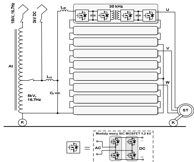
Rys. 1. Schemat proponowanego rozwiązania hybrydowego transformatora energoelektronicznego z autotransformatorem obniżającym napięcie sieci trakcyjnej
