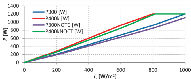
Rys. 10. Wpływ temperatury na moc czynną, generowaną przez mikroelektrownię PV o mocy znamionowej P_n = 1200 W, w funkcji stałej wartości natężenia promieniowania słonecznego I_x
