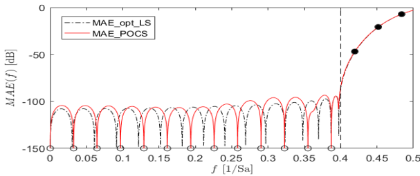
Rys. 1. Moduł zespolonego błędu aproksymacji filtru FD optymalnego w sensie pasmowego kryterium LS (linia przerywana) dla N=31 , f_a = 0.4 , d=0.25 oraz odpowiadającego mu filtru DFT-VFD optymalnego dla p=3 [1]
