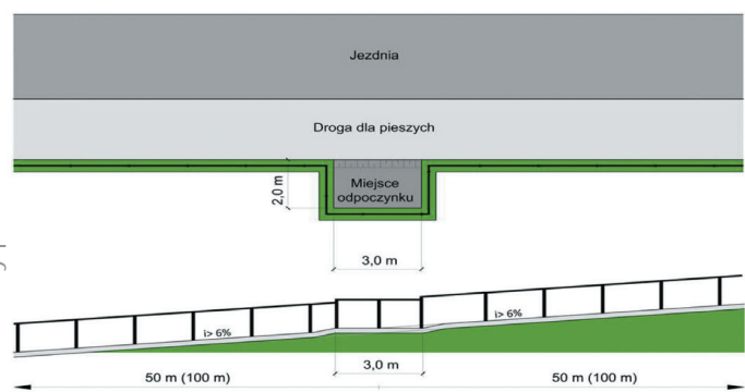
Rys. 23. Przykład lokalizacji miejsca odpoczynku dla osób o szczególnych potrzebach na drodze dla pieszych usytuowanych przy drodze o pochyleniu większym od 6% Źródło: opracowanie własne
