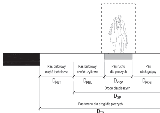
Rys. 16. Schemat przekroju poprzecznego drogi dla pieszych uwzględniający pas terenu przy drodze niezbędny do wybudowania drogi dla pieszych w obszarze zamiejscowym
