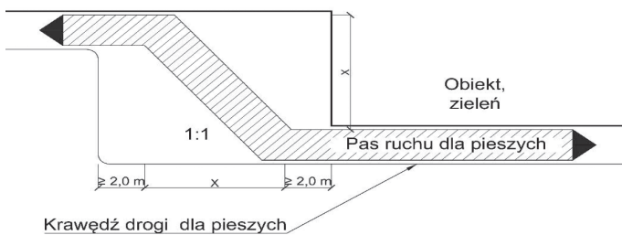
Rys. 22. Schemat placu do zmiany przebiegu pasa ruchu lub drogi dla pieszych w miejscu załamania lub uskoku trasy
