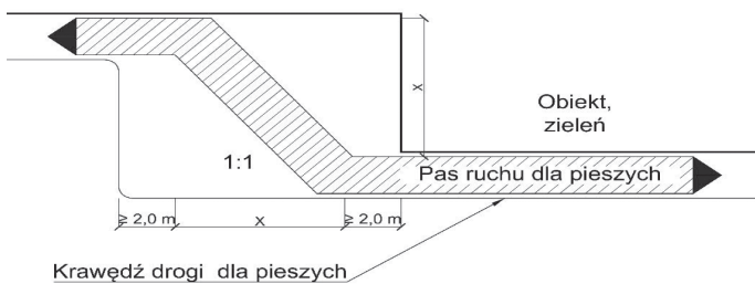
Rys. 22. Schemat placu do zmiany przebiegu pasa ruchu lub drogi dla pieszych w miejscu załamania lub uskoku trasy Źródło: opracowanie własne
