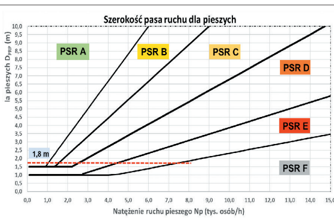
Rys. 21. Pas ruchu dla pieszych – wykres służący do ustalania szerokości pasa w zależności od natężenia ruchu pieszego i przyjętego poziomu warunków ruchu pieszego
