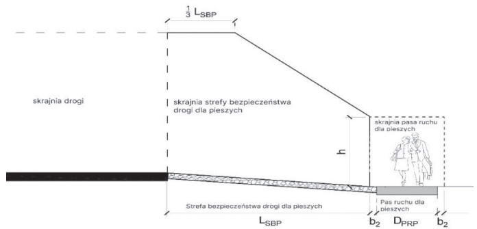
Rys. 11. Usytuowanie drogi dla pieszych wzdłuż drogi zamiejscowej lub ulicy poza strefą bezpieczeństwa drogi
