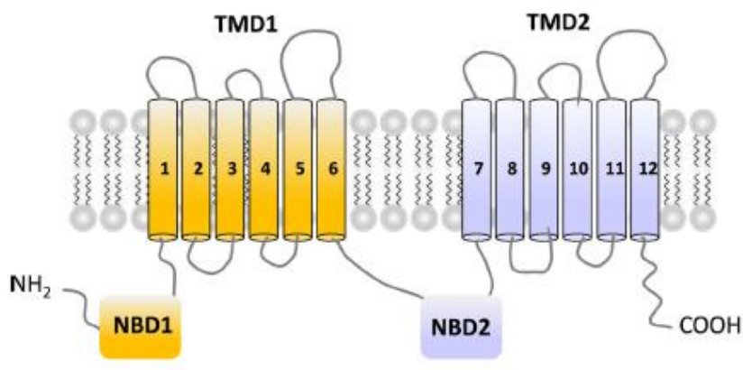
Rys. 1. 2. Topologia transportera Cdr1p należącego do rodziny ABC [18]
