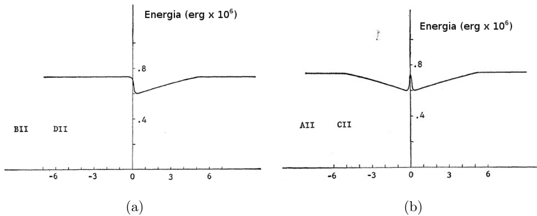
Rysunek 2.12: Rozkład energii granicy domenowej 90° w pobliżu inkluzji [72].
