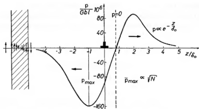
Rysunek 2.10: Oddziaływanie dyslokacji liniowej na 180° granicę domen magnetycznych [54]. W zależności od zwrotu wektora Burgersa dyslokacja liniowa przyciąga lub odpycha granicę.
