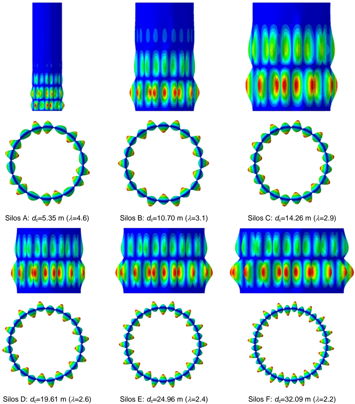
Rys. 6.58. Pierwsza postać wybojzeniowa silosów A–F o rozstawie żeber d_s=0.7 m
