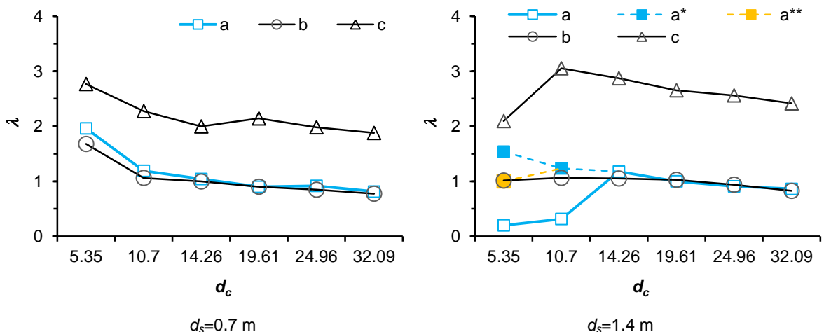
Rys. 6.82. Dopuszczalny mnożnik obciążenia \lambda dla silosów A–F wyznaczony na podstawie: a) [PN-EN 1993-4-1], a*) wg proponowanej metody i współczynnika k_{\alpha x}=9.3 , a**) wg proponowanej metody i normowego współczynnika k_{\alpha x}=7.4 , b) liniowej analizy wyboczeniowej silosu obciążonego tarcieniem ( \alpha_{x,GNIA^*}=0.4 ), c) liniowej analizy wyboczeniowej silosu z obciążeniem stycznym i normalnym ( \alpha_{x,GNIA^*}=0.4 )
