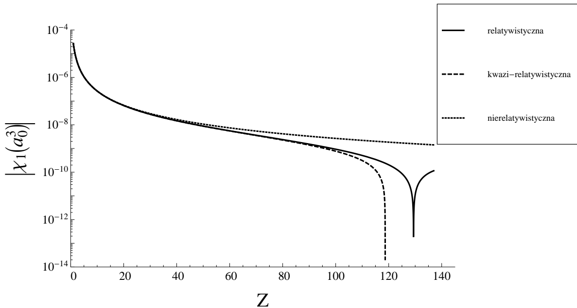
Rys. 32: Wartość bezwzględna statycznej magnetyzowalności dipolowej \chi_1 dla atomu jednoelektronowego w stanie podstawowym jako funkcja liczby atomowej Z . Porównanie formuły relatywistycznej (10.32), kwazi-relatywistycznej (10.37) i nierelatywistycznej (10.42).
