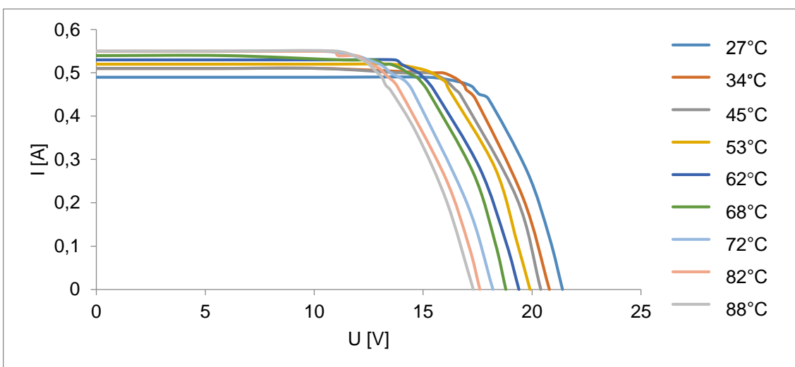
Rysunek 3. Porównanie charakterystyk prądowo-napięciowych Układu 1 dla różnych wartości temperatury pracy Modułu 4
