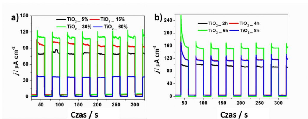
Rysunek 25. Zmiany gęstości generowanego fotoprądu podczas oświetlania fotoanod otrzymanych w różnych warunkach procesu anodyzacji: a) w zależności od ilości wody w elektrolicie oraz b) w zależności od czasu anodyzacji.
