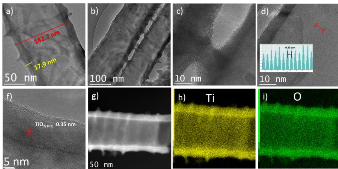
Rysunek 73. Zdjęcia TEM niemodyfikowanych nanorurek ditlenku tytanu.
