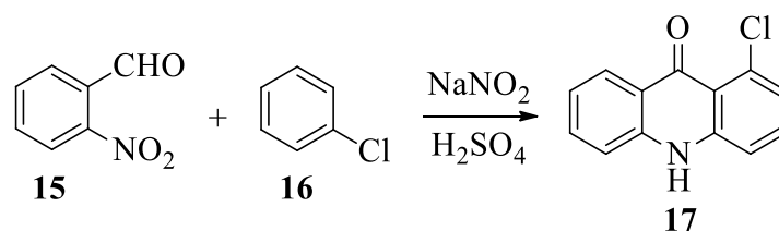
Schemat 3. Otrzymywanie akrydonu ( 17 ) metodą Lehmstedta-Tanasescu [8].
