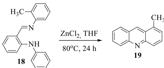
Schemat 4. Synteza pochodnych akrydyny ( 19 ) oparta na reakcji cyklizacji zasady Schiffa o -aryloaminofenyłu w obecności ZnCl_2 [11].
