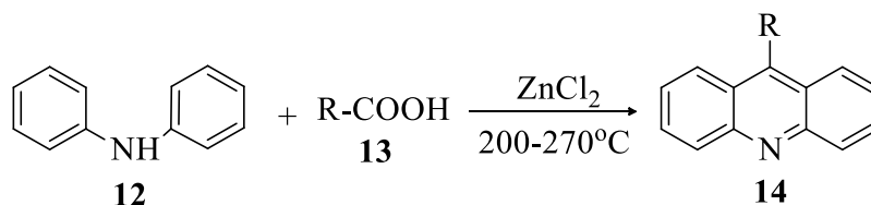
Schemat 2. Otrzymywanie pochodnych akrydyny ( 14 ) metodą Brenthseny [7].
