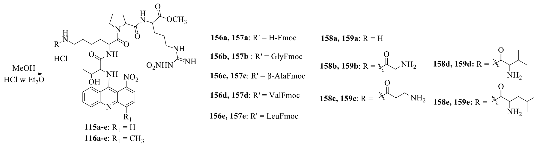
Schemat 22. Synteza pochodnych 1-nitro ( 115a-e )/4-metylo-nitroakrydiny ( 116a-e ) z analogami tuftsyny.
