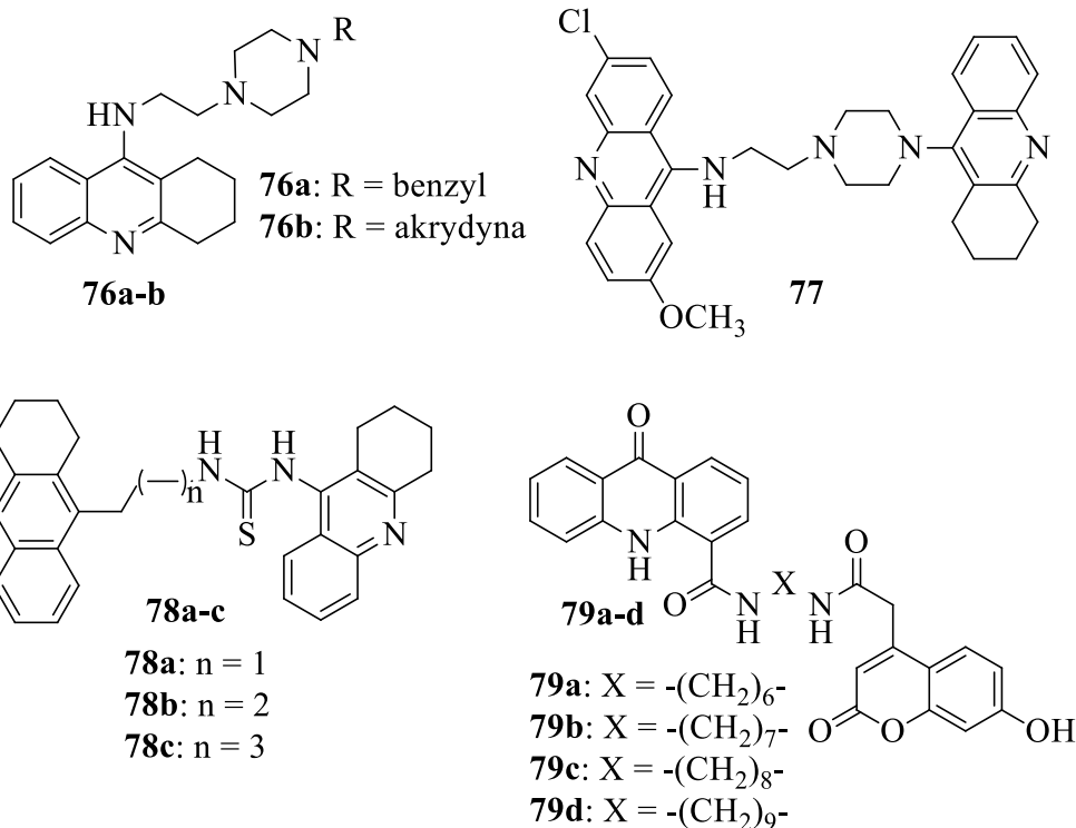
Rys. 4. Struktury chemiczne hybrid akrydyny z takryną ( 76a-b , 77 , 78a-c ) [41] oraz akrydonu z kumaryną ( 79a-d ) [42].
