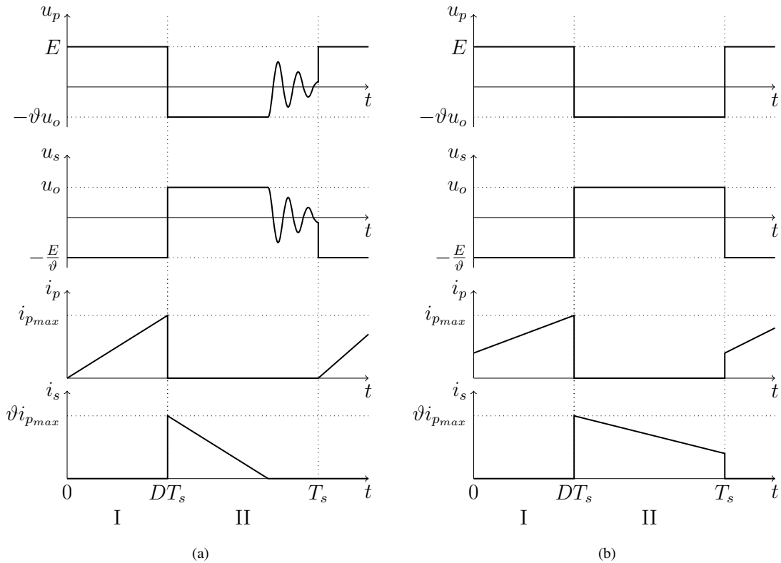
Rys. 2.2: Przebiegi prądów i napięć w przekształtniku dwutaktowym pracującym w trybie: a)przewodzenia przerywanego; b) przewodzenia ciągłego.
