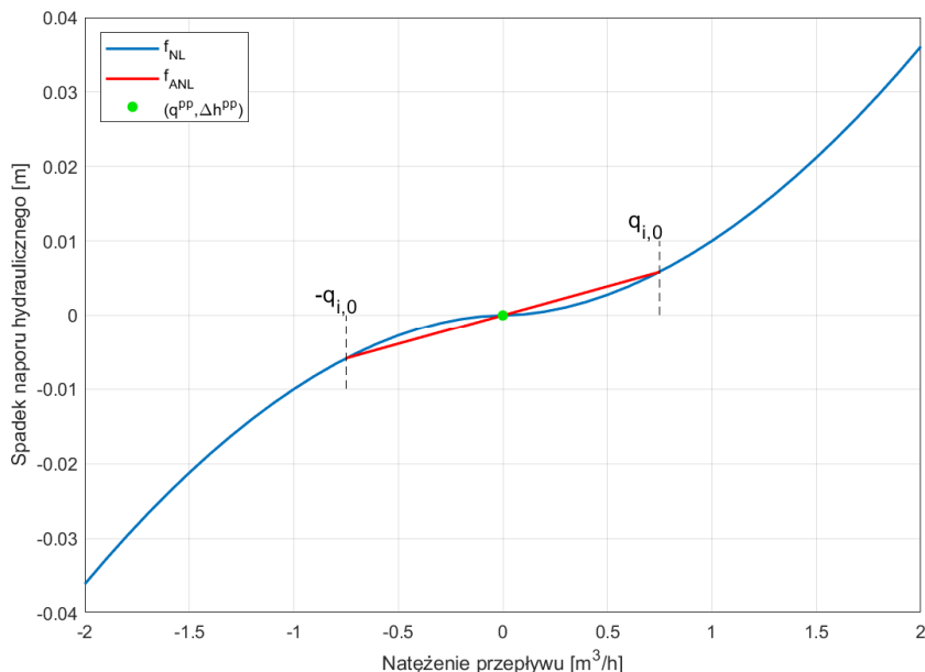
Rysunek 5.8. Ilustracja linearyzacji jednodzinkowej charakterystyki ruociągu dla przypadku, gdy |q_i^{pp}(t_n + k | t_n)| \leq q_{i,0} .
