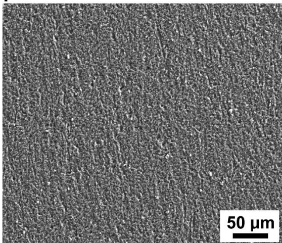
Rys. 70. Mikrografie SEM przedstawiające topografię powierzchni stopu aluminium AA1050 po polaryzacji anodowej do +8 V vs Ag|Ag 2 O stosowanej w trakcie pomiarów LSV + DEIS. Powiększenie: 250x [640].
