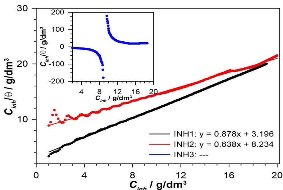
Rys. 117. Izotermi adsorpcji Langmuira wyznaczone na podstawie pomiarów g-DEIS dla stopu aluminium AA5754 eksponowanego w buforze wodorowęglanowym ( \text{pH} = 11 ) z dodatkiem badanych ekstraktów inhibitorów korozji [798].
