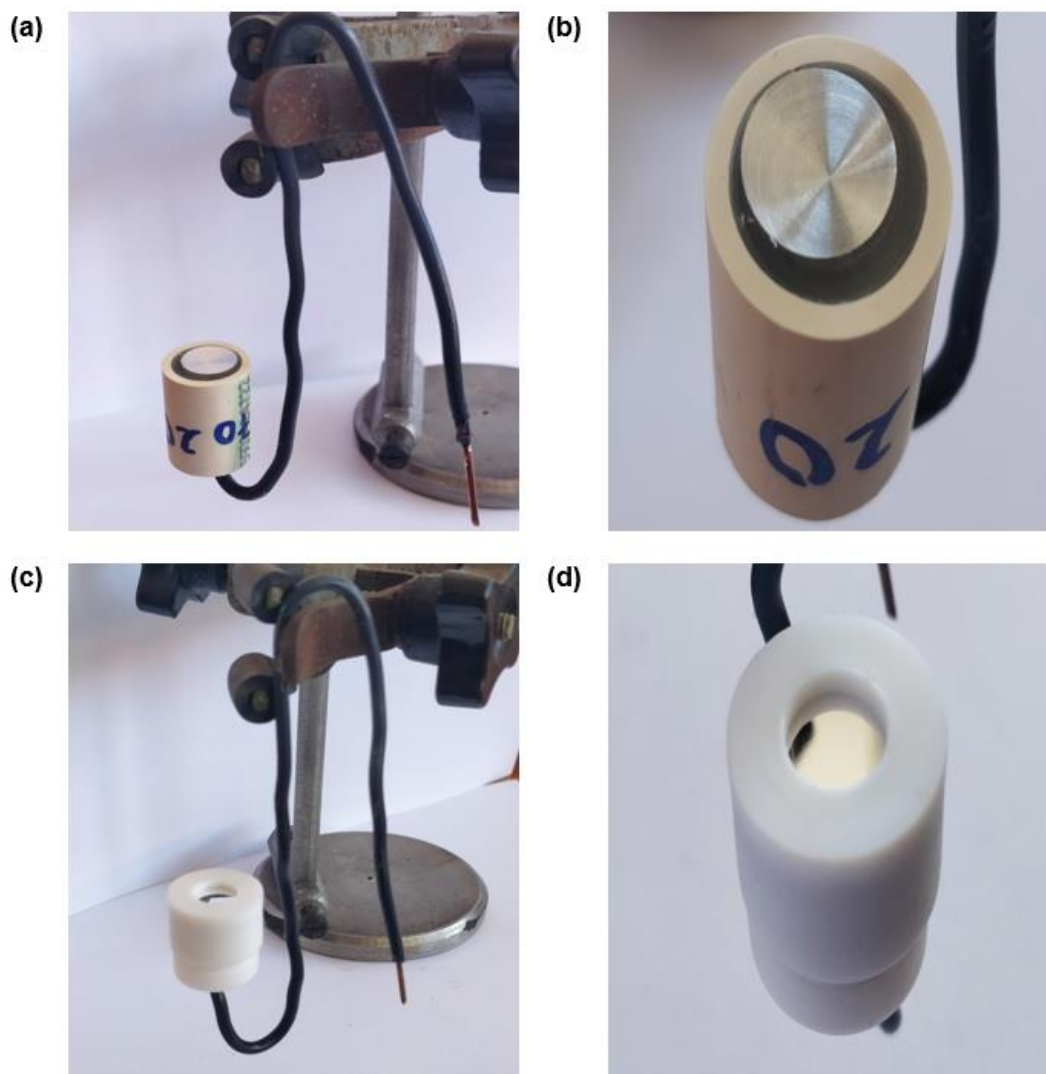
Rys. 23. Konstrukcja próbek stosowanych do badań elektrochemicznych: (a) i (b) zatapianych w żywicy chemoutwardzalnej, (c) i (d) montowanych w uchwytach z teflonu.
