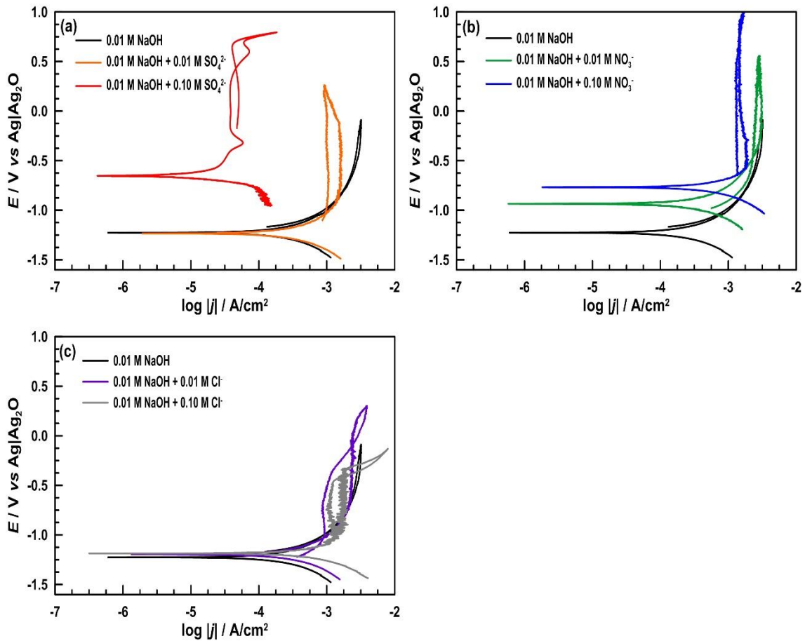
Rys. 85. Krzywe polaryzacji cyklicznej E = f(\log |j|) zarejestrowane dla stopu aluminium AA2024 eksponowanego w 0.01 mol/dm 3 roztworze NaOH z dodatkiem jonów: (a) SO_4^{2-} , (b) NO_3^- , (c) Cl^- . Zakres polaryzacji: od -0.25 V vs E_{OCP} do +1.50 V vs Ag|Ag 2 O. Szybkość zmian potencjału w czasie: 1 mV/s. Graniczna gęstość prądu: 10 mA/cm 2 .
