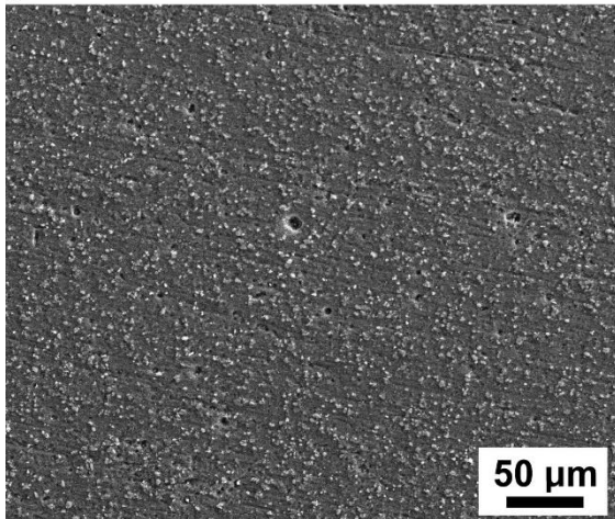
Rys. 69. Mikrografie SEM przedstawiające topografię powierzchni stopu aluminium AA1050 po 1.5 h ekspozycji w środowiskach zasadowych o pH 14 – 8.5 w warunkach samo-korozji. Powiększenie: 250x [640].
