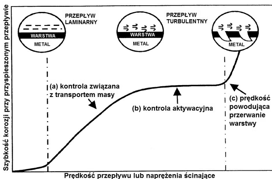
Rys. 14. Wpływ prędkości przepływu środowiska na szybkość korozji materiałów metalicznych [167].
