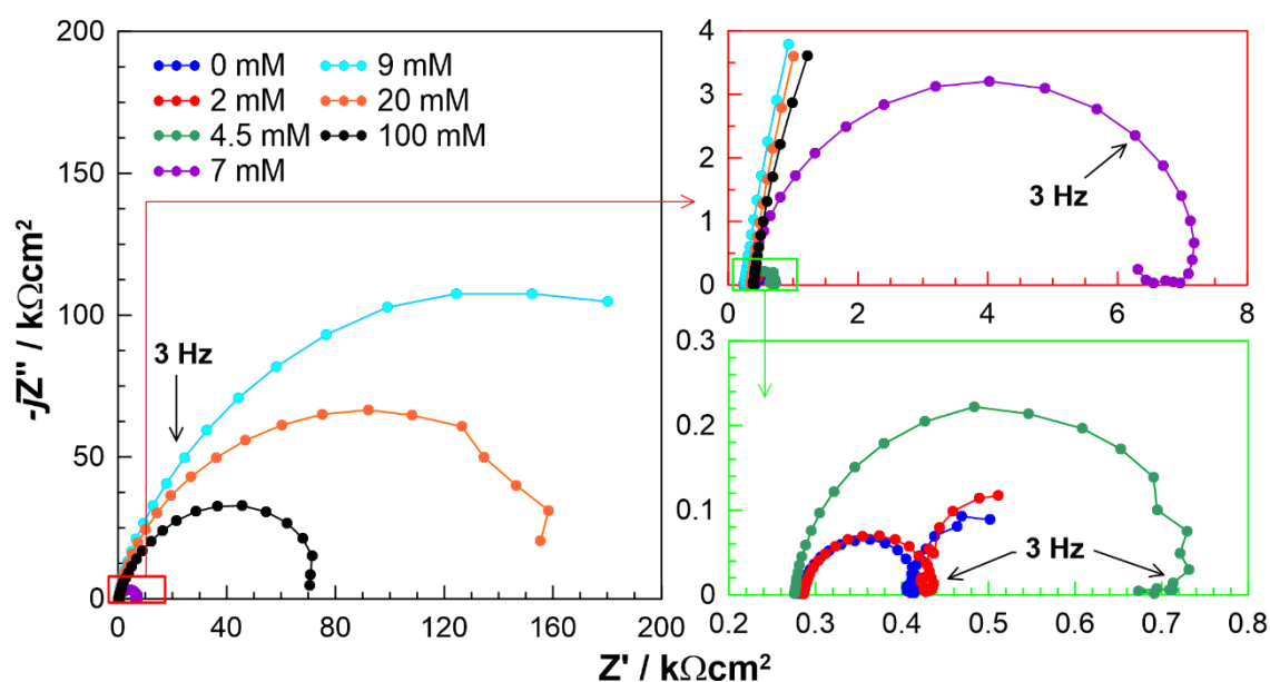
Rys. 99. Widma impedancyjne EIS w projekcji Nyquista zarejestrowane dla stopu aluminium AA5754 eksponowanego w buforze wodorowęglanowym ( \text{pH} = 11 ) z dodatkiem różnych stężeń kwasu cytrynowego. Zakres częstotliwości: od 10.0 \text{ kHz} do 0.1 \text{ Hz} . Amplituda pik-pik sygnału pobudzenia: 15 \text{ mV} . Pomiary EIS realizowano w trybie potencjostatycznym przy ustabilizowanej wartości potencjału korozyjnego. Układ przed pomiarem kondycjonowano przez 30 \text{ min} [743].
