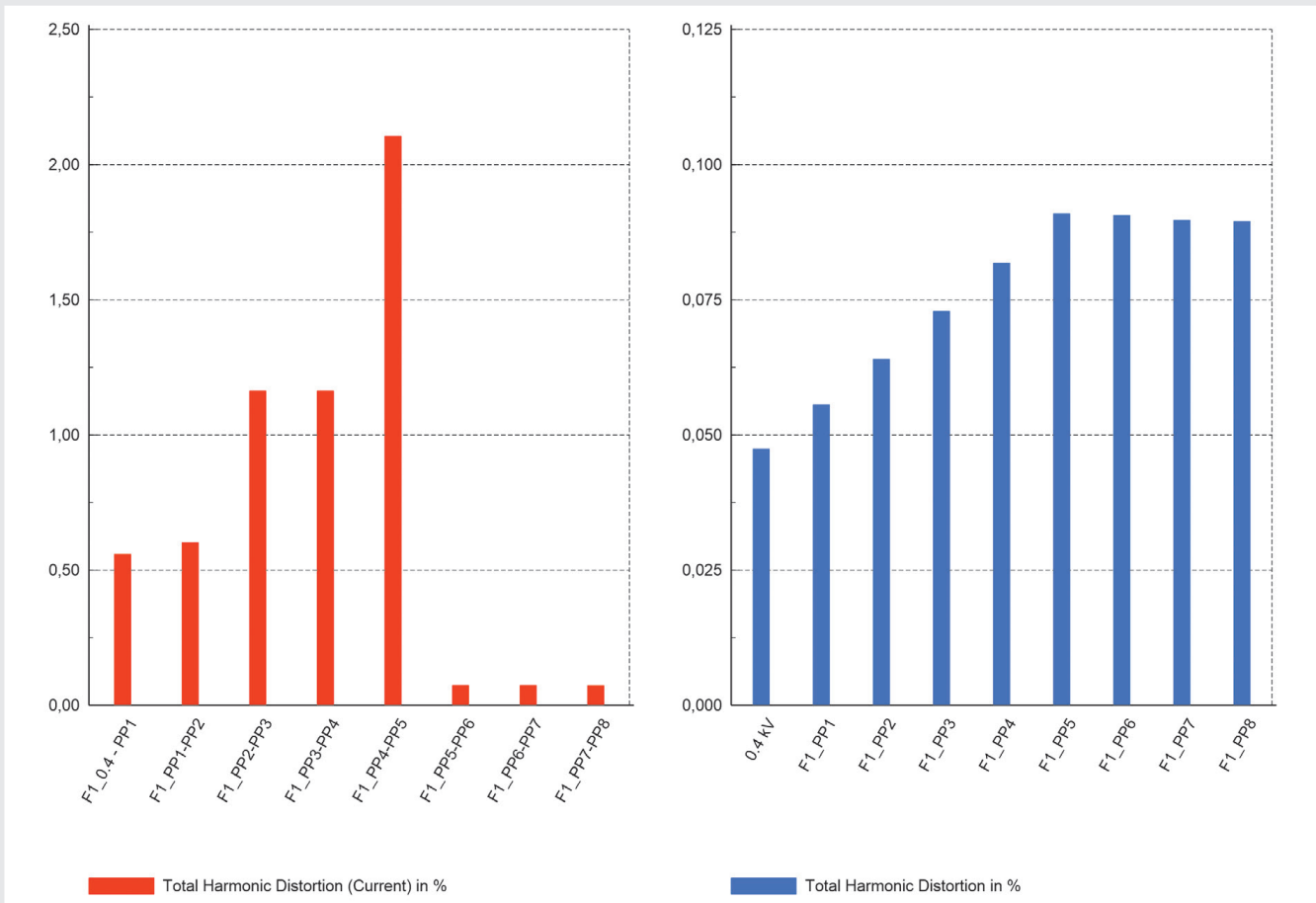
Rys. 9. Współczynnik THD prądu w liniach i THD napięcia na szynach obwodu z mikrogeneracją o P = 16,2 kW
