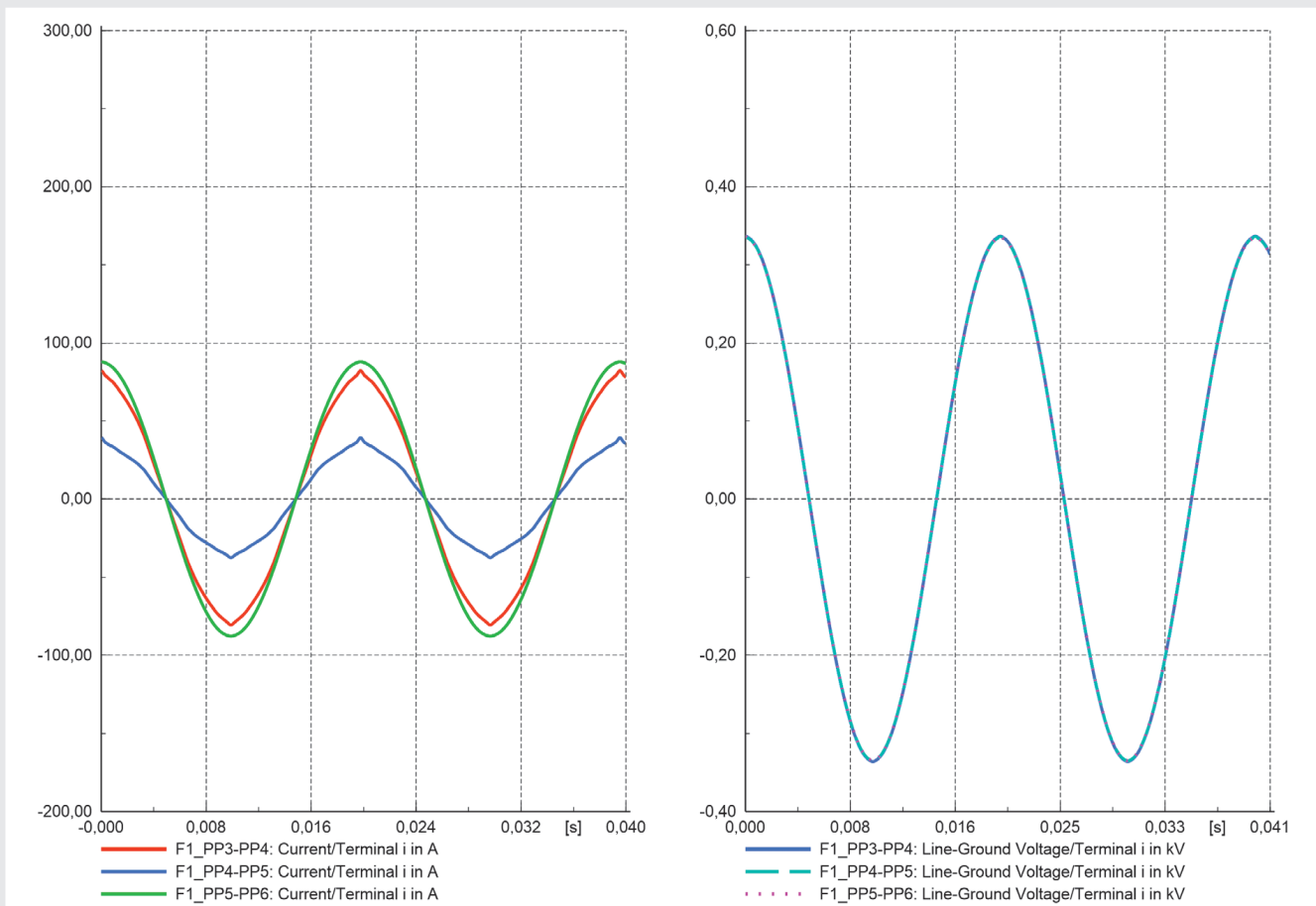
Rys. 11. Kształt napięcia i prądu w liniach przed i za punktem przyłączenia mikroźródła o P = 26,4 kW
