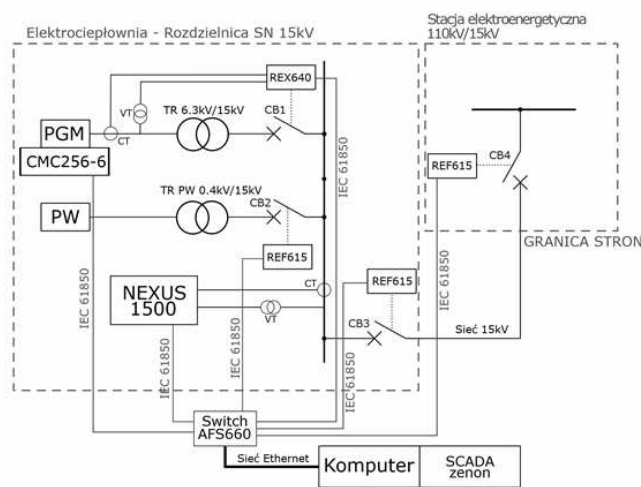
Rys. 5. Graficzne przedstawienie struktury zamodelowanej sieci (PGM – moduł wytwarzania energii, PW – potrzeby własne)
