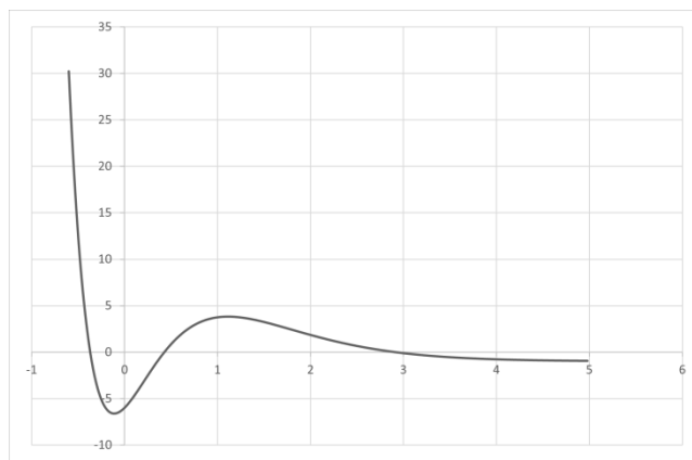
Rys. 5. Wykres funkcji f(x) = (40x^2 - 5)e^{-2x} - 1
