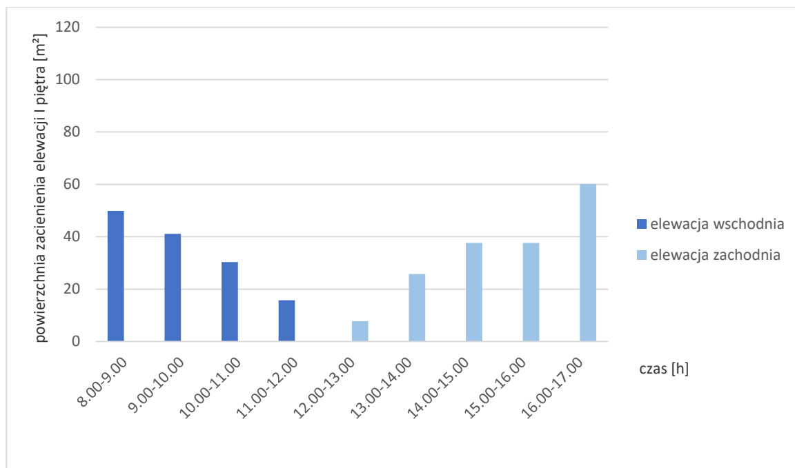
Rysunek 63. Powierzchnia zacielenia elewacji na wysokości I piętra przez szpaler drzew zlokalizowany w odległości 2 m od zabudowy w modelu ulicy na osi północ-południe z zabudową wysoką o H/W \leq 0,6 w dniu 7 czerwca w godzinach 8.00–17.00
