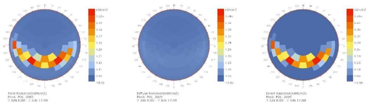
Rysunek 31. Schemat ilustrujący nieboskłon z lokalizacją promieniowania słonecznego całkowitego, rozproszonego i bezpośredniego w wybranej lokalizacji (Płock) w dniu 7 czerwca w godzinach 8.00-17.00 Źródło: Opracowanie własne na podstawie plików pogodowych EPW: https://www.energyplus.net/weather-download/europe_wmo_region_6/POL//POL_Plock.123600_IMGW/all (dostęp: 25.03.2020).
