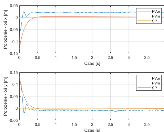
Rys. 5. Odpowiedź skokowa rzeczywistego układu regulacji i jego modelu Fig. 5. The step responses of the platform model and the platform
