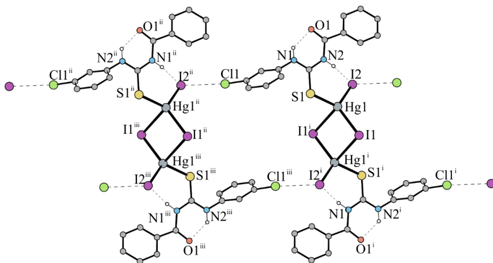
Rys. 214. Oddziaływania halogenowe Cl \cdots I występujące w strukturze Hg^{13} . Wiązania C-H pominięto dla przejrzystości. Operacje symetrii: (i) -x, 1 - y, -z ; (ii) x, 1 + y, z ; (iii) -x, 2 - y, -z .
