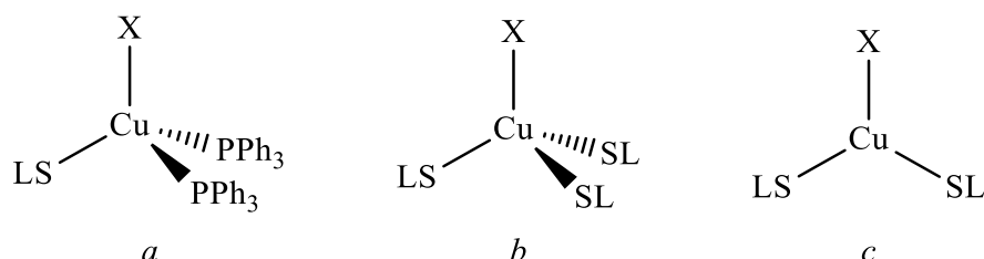
Rys. 20. Typy jednordzeniowych związków kompleksowych miedzi z 1-ac-3-monotem (LS), X: halogen.
