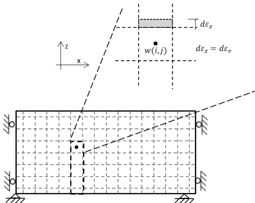
Rys. 6.9. Schemat wyznaczania odkształceń liniowych dla jednowymiarowego stanu odkształcenia
