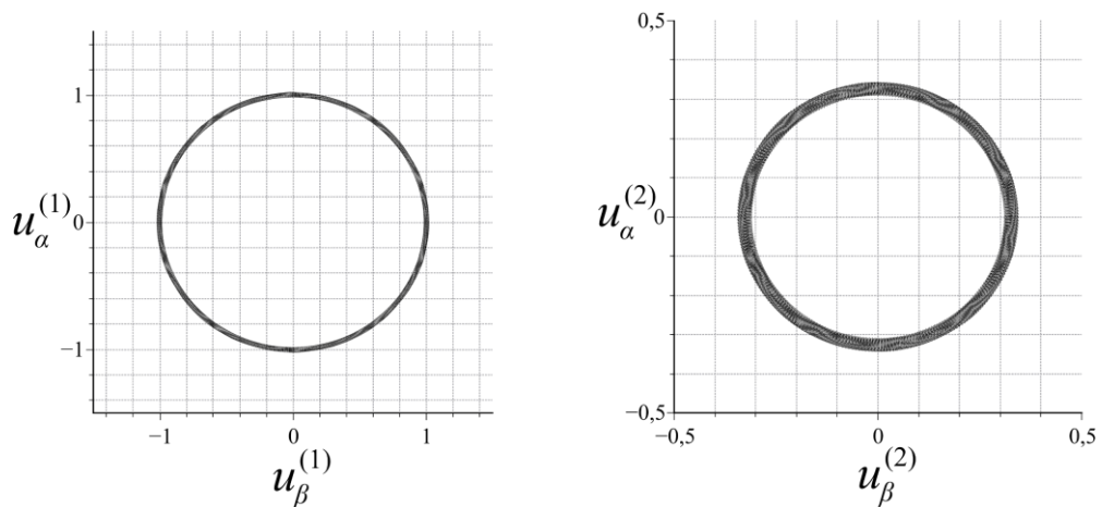
Rys. 9.2. Hodografy wektorów przestrzennych napięcia obciążenia w układach współrzędnych \alpha^{(1)} - \beta^{(1)} i \alpha^{(2)} - \beta^{(2)} dla metody wykorzystującej osiem wektorów aktywnych
