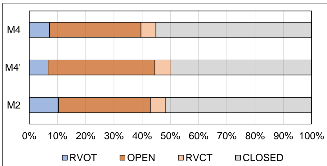
Rys. 8.20. Udział procentowy poszczególnych faz cyklu pracy badanych modeli protez, gdzie RVOT – czas szybkiego otwierania protezy, OPEN – czas fazy pełnego otwarcia i powolnego zamykania, RVCT – czas szybkiego zamykania, CLOSED – czas, podczas którego proteza jest zamknięta.
