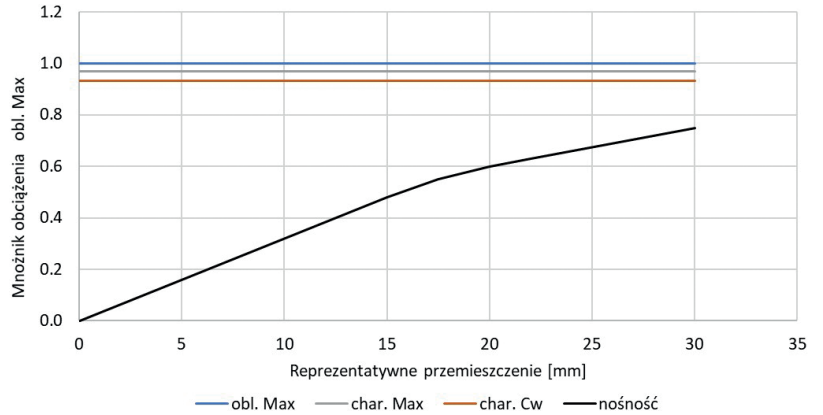
Rys. 13 Wynik analizy węzła nr 2201. Wykres siła-przemieszczenie (mnożnik dla obl. siły max w linii dla Cw+kl A)
