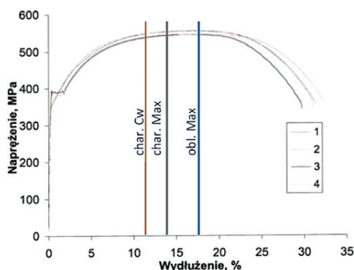
Rys. 16. Stan maksymalnych odkształceń materiału węzła 2201 naniesiony na wynik testu jednoosiowego rozciągania
