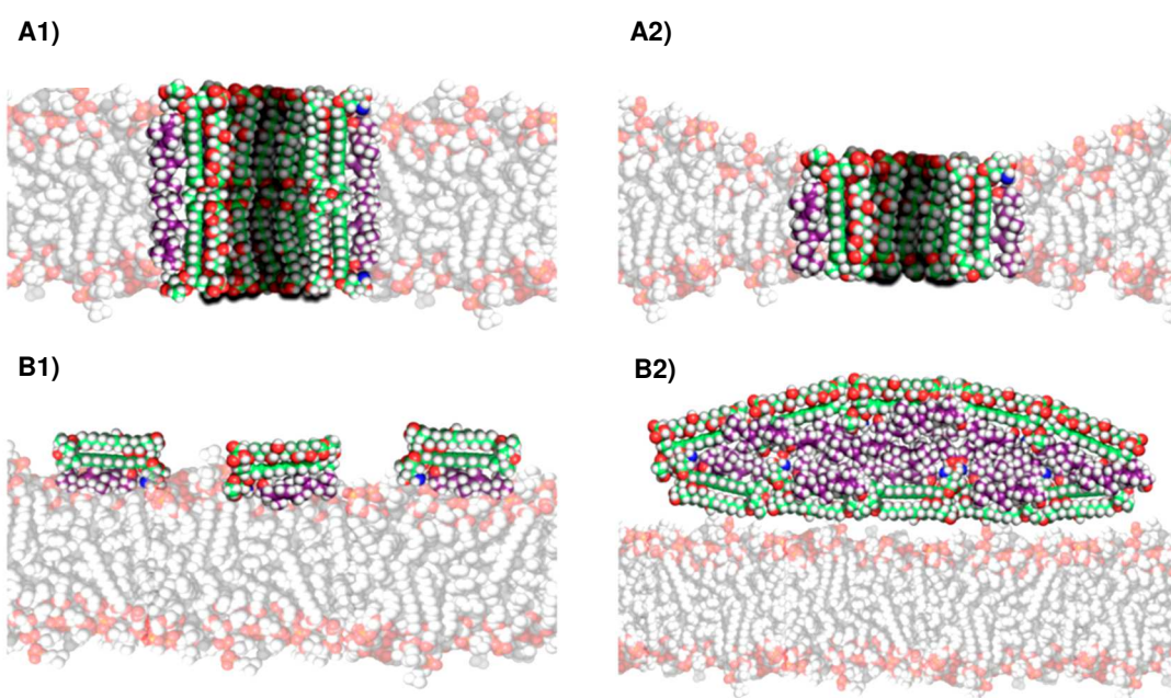
Rys. II. 1.2. Schematy zaproponowanych modeli oddziaływań AmB-ergosterol: A1) kanał jonowy, A2) półkanał jonowy, B1) wyłapywanie steroli przez cząsteczki AmB zaadsorbowane na powierzchni błony, B2) sterolowa gąbka [26].
