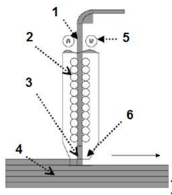
Rys. 4. Schemat procesu wydruku w technologii FDM: 1 – filament; 2 – grzałki; 3 – materiał modelowy; 4 – budowany model; 5 – rolki; 6 – dysza - źródło [62]
