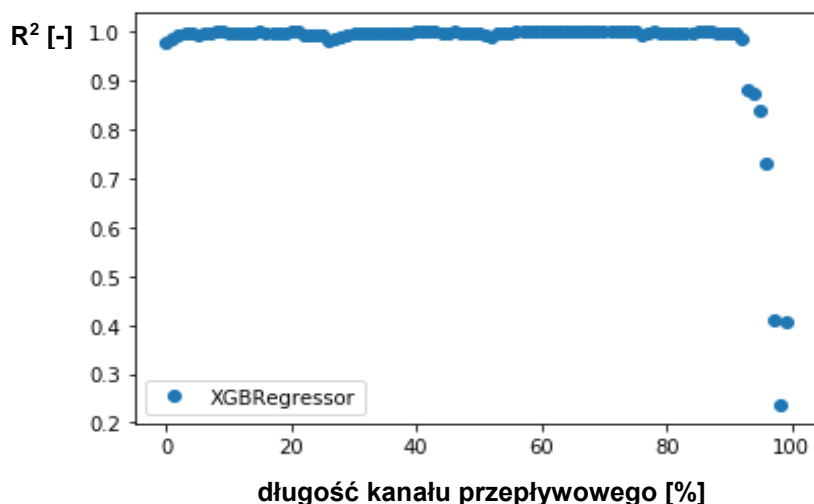
Rys. 4.6. Wynik testu wzdłuż osi turbiny – wartość współczynnika determinacji ( R^2 ) osiągnięta przez model XGBRegressor na kolejnych podzbiorach zbioru testowego.
