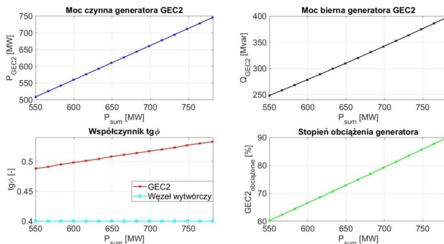
Rys. 6.11. Parametry pracy generatora GEC2 przy utrzymywaniu przez przekształtnik stałej stałego współczynnika \text{tg}\phi na szynach węzła wytwórczego
