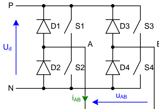
Rys. 3.1. Struktura falownika jednofazowego [4]
