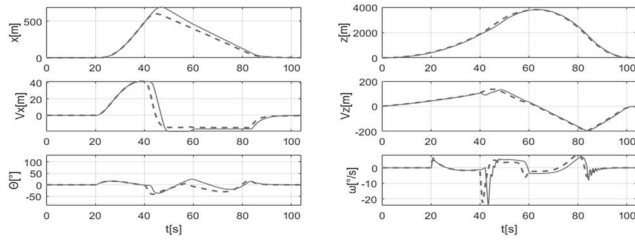
Rys. 7. Porównanie trajektorii stanu dla symulacji w środowisku MATLAB (linia przerywana) oraz symulacji w pętli sprzętowej HIL (linia ciągła)
