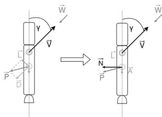
Rys. 2. Przekształcenie siły oporu powietrza D oraz siły nośnej L na siłę aerodynamiczną o kierunku zgodnym z osią wzdluzną A oraz siłę o kierunku prostopadłym do tej osi N
