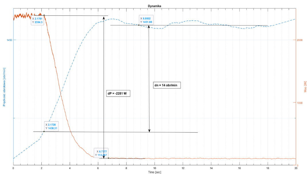
Rys. 5 Zmiany P_e , n = f(t) , olej napędowy VERVA ON gatunek B, a) etap I, b) etap II. (uśrednione wyniki pięciu serii pomiarowych)
