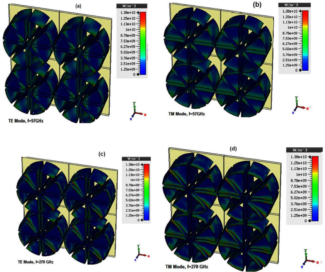
Figure 6. The power loss density at (a) f=57\text{ GHz} , TE mode (b) f=57\text{ GHz} , TM mode (c) f=270\text{ GHz} , TE mode and (d) f=270\text{ GHz} , TE mode.
