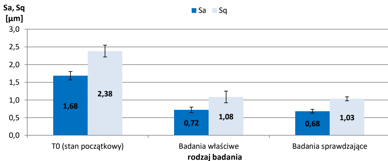
Rysunek 70. Wartości średnie parametrów Sa oraz Sq po poszczególnych etapach badań eksperymentalnych docierania jednostronnego ceramiki technicznej Al_2O_3
