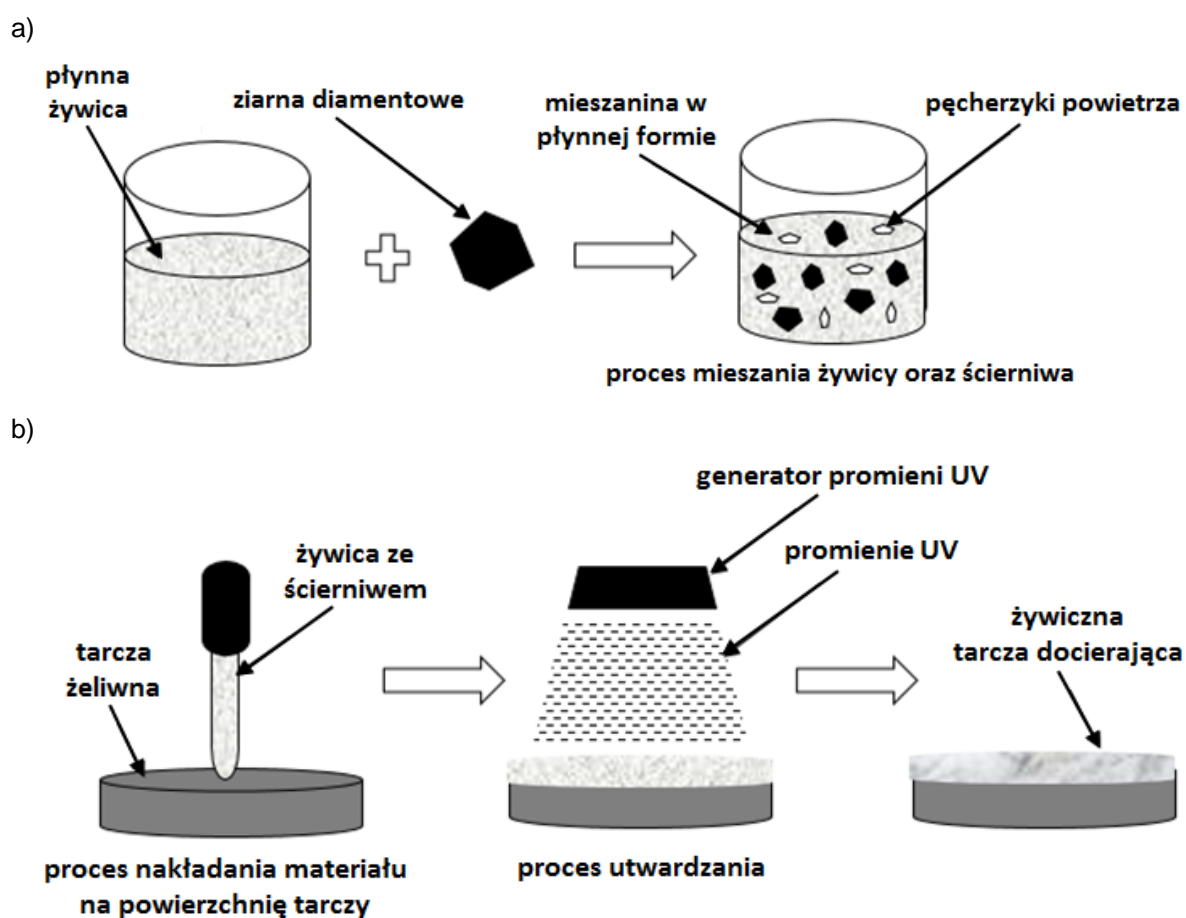
Rysunek 18. Sposób wytwarzania tarczy docierającej o spoiwie żywicznym: a) przygotowanie materiału w postaci płynnej żywicy oraz ścierniwa; b) proces nakładania materiału i jego utwardzania (Huang, Guo and Marinescu, 2015; Guo, Zhang, Chen, et al., 2019; Deja et al., 2021)
