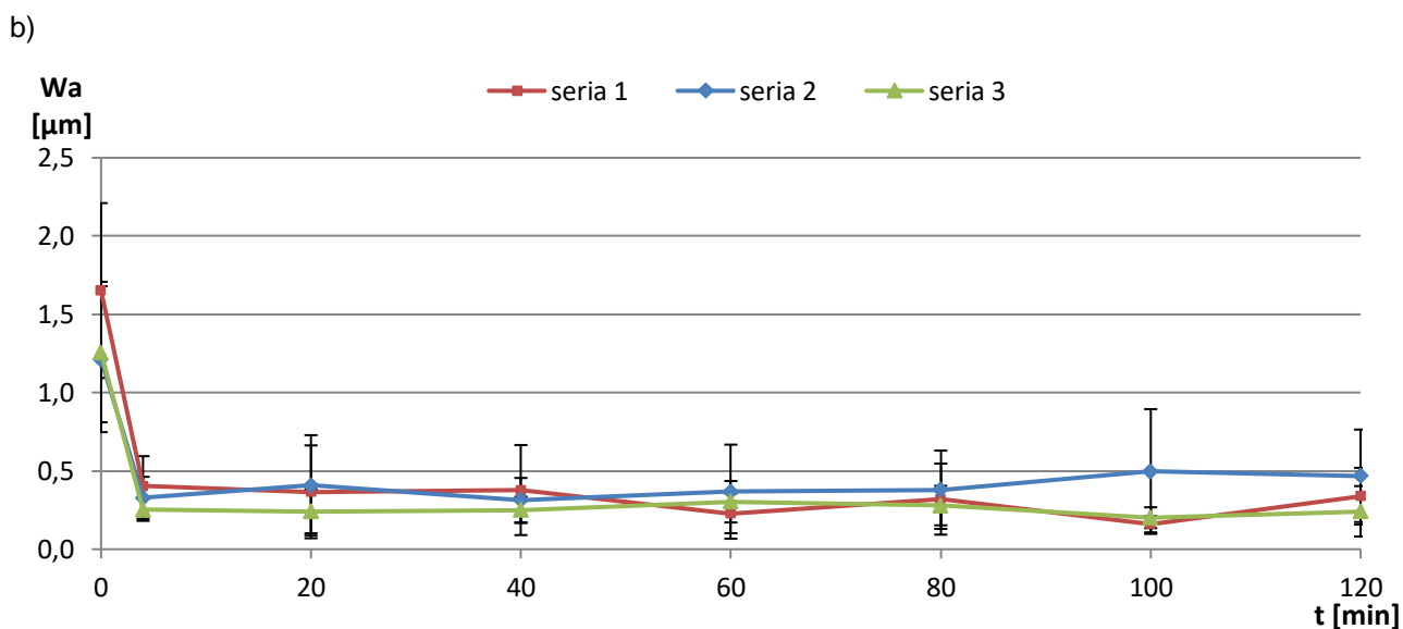
Rysunek 65. Wartości parametrów chropowatości Ra (a) oraz falistości Wa (b) PO uzyskane podczas badań sprawdzających docierania jednostronnego ceramiki technicznej Al_2O_3
