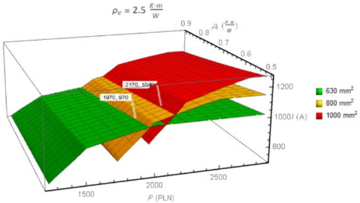
Rysunek 33. Obciążalność prądowa kabli WN (630 mm 2 , 800 mm 2 i 1000 mm 2 ) w konfiguracji płaskiej jako funkcja kosztów instalacji kabla oraz rezystywności cieplnej wypełnienia kontrolowanego i ziemi rodzimej: (a) \rho_e = 1,0 (K·m)/W; (b) \rho_e = 1,5 (K·m)/W; (c) \rho_e = 2,0 (K·m)/W; (d) \rho_e = 2,5 (K·m)/W.
