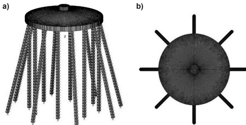
Rys. 4. Model fundamentu podpory a) widok ogólny b) widok z góry
