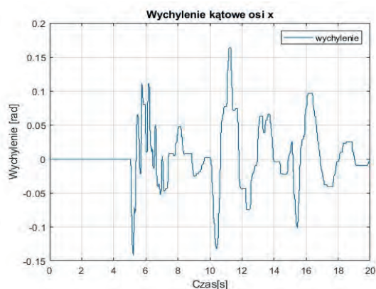
Rys. 13. Wychylenie kątowne dla osi x z klasycznym regulatorem PID
