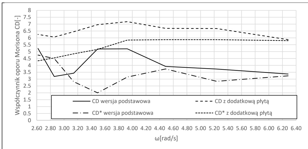
Rysunek 68 Skorygowane wartości współczynnika równania Morisona dla wersji podstawowej oraz wersji z dodatkową płytą tłumiącą.
