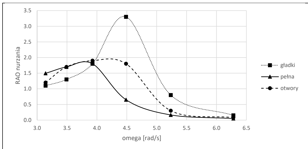
Rysunek 48 Wartości RAO nurzania funkcji przeniesienia obliczone w programie ANSYS AQWA rozszerzonym o dodatkowy współczynnik tłumienia liniowego.
