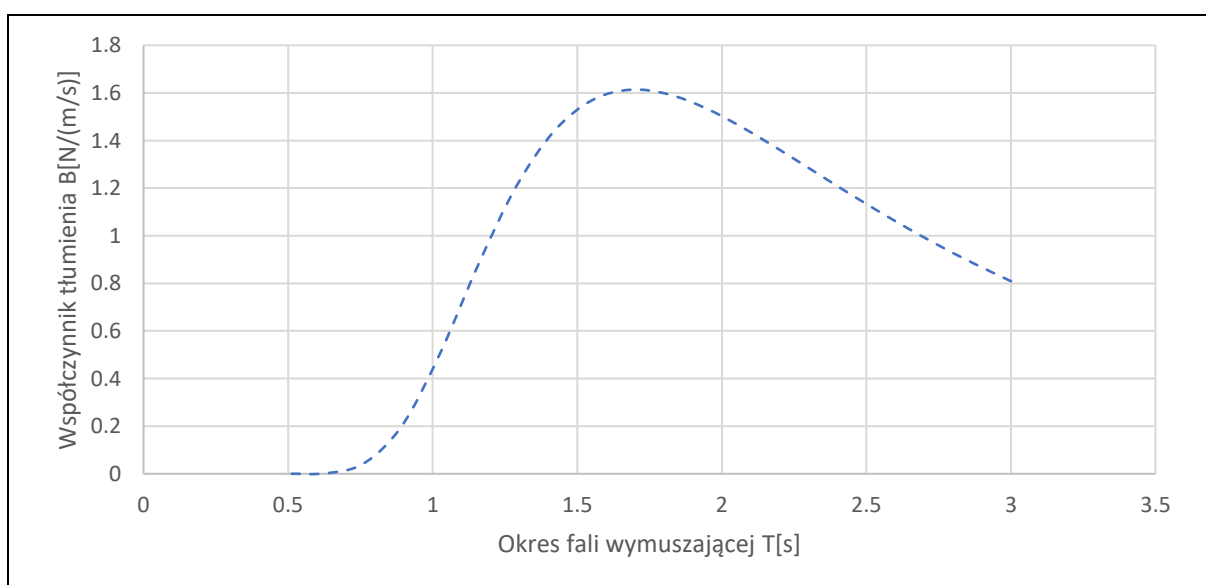
Rysunek 46 Współczynnik tłumienia dla cylindra z płytą z otworami
