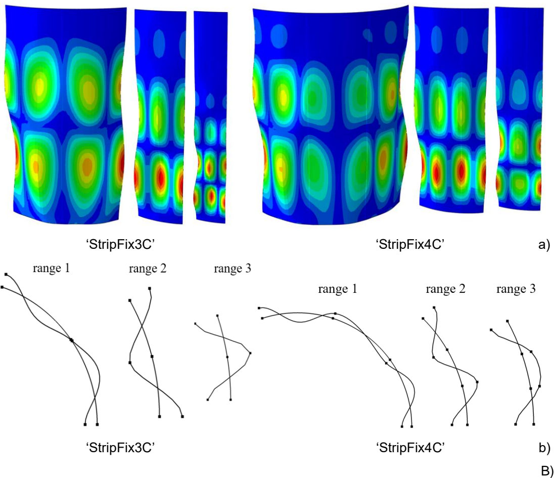
Rys. 5.17: Liniowe analizy wyoboczenia LBA dla silosu S1600 (rys. 5.2c) obciążonego naporem stycznym (przypadek obciążenia „V”): A) współczynnik obciążenia wyoboczeniowego \lambda w zależności od liczby słupów n dla modeli: a) model ‘3D’-‘ortho-beam’ z dostosowanym przekrojem poprzecznym słupa do rozkładu sił normalnych w słupie uwzględniający mimośród w stosunku do ściany (b) ‘StripFix3C’, c) ‘StripFix4C’, d) ‘EC3A’ [4], e) ‘EC3B’ [4] and f) ‘EC3B+’ [5], B) postaci wyoboczeniowe modelu całego silosu ‘3D’ w zakresach ‘1’-‘3’: a) widok 3D i b) przekrój poziomy oraz C) postaci wyoboczeniowe modeli segmentów silosu ‘StripFix3C’ i ‘StripFix4C’ (a) widok 3D i b) przekrój poziomy).
