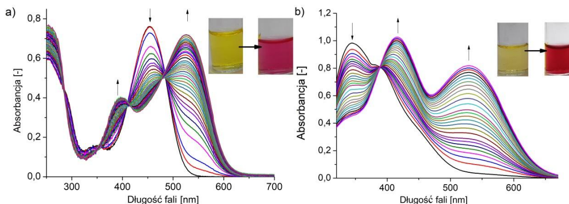
Rys. 4.17. Zmiany w widmie absorpcyjnym podczas miareczkowania roztworem kwasu para -toluenosulfonowego (TosOH): a) związku BiF-19-p-OH ( c = 2,66 \cdot 10^{-5} \text{ mol/dm}^3 ); c_{\text{TosOH}} = 0-1,35 \cdot 10^{-4} \text{ mol/dm}^3 , b) związku BiF-19-o-OH ( c = 6,91 \cdot 10^{-5} \text{ mol/dm}^3 ); c_{\text{TosOH}} = 0-1,23 \cdot 10^{-3} \text{ mol/dm}^3 w acetonitrylu
