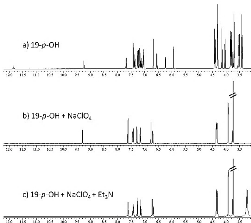
Rys. 4.56. Widma ^1\text{H} NMR zarejestrowane dla związku 19\text{-}p\text{-OH} ( c = 1,3 \cdot 10^{-3} \text{ mol/dm}^3 ) z chloranem(VII) sodu (równomolowa ilość) oraz z dodatkiem trietyloaminy w acetonitrylu- \text{d}_3
