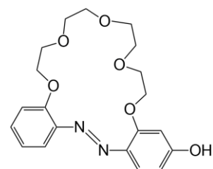
19-p-OH
