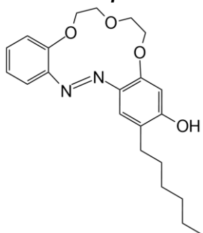
C6-13-p-OH
