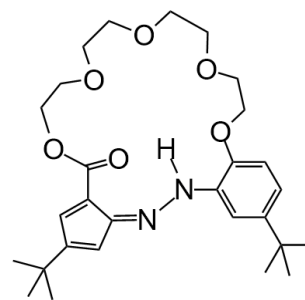
t-Bu-20-ester
