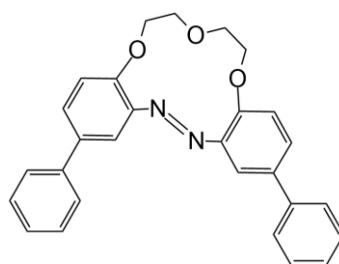
BiF-13-Azo
