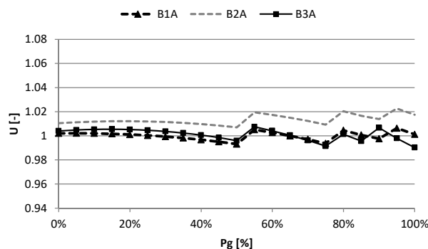
Rys. 6. Zmienność napięć przy stałej wartości napięcia zadane.
