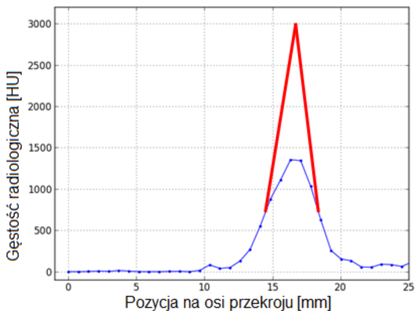
Rys. 5.3 Niebieska linia – gęstość radiologiczna przekroju zdjęcia TK w przekątnej próbki zaznaczonej na Rys. 5.2. Czerwona linia – gęstość radiologiczna wirtualnej próbki. (opracowanie własne).
