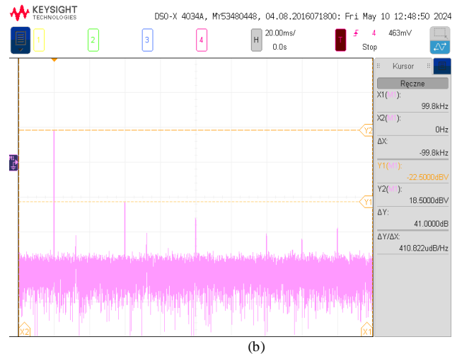
Fig. 8. Spectrum for TPA 3255 (10% duty cycle) (a) 4 kHz (b) 8 kHz (c) 7 kHz (d) 17 kHz (e) 16 kHz (f) 30 kHz
