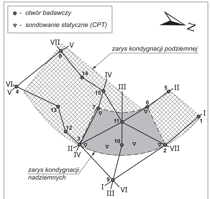
Rys. 5 Usytuowanie wiercni badawczych i sondowań statycznych pod budynek PPPL
