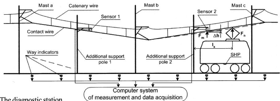
Fig. 5. Idea of the vertical force measurement on checking section Rys. 5. Koncepcja sieciowego pręśla pomiarowego
