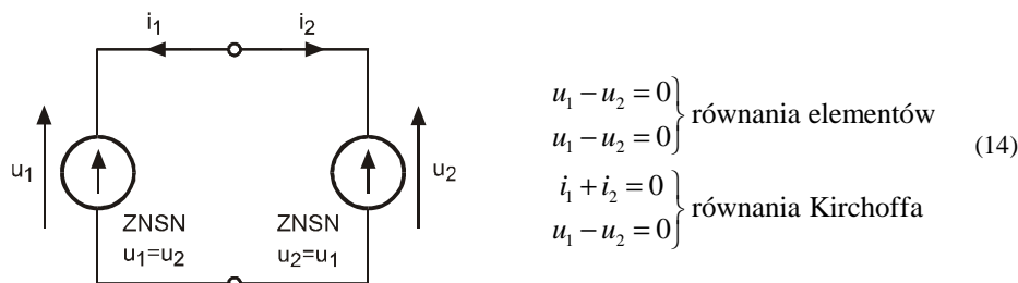
Rys. 1. Układ napięciowych źródeł sterowanych
