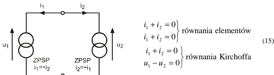
Rys. 2. Układ prądowych źródeł sterowanych
