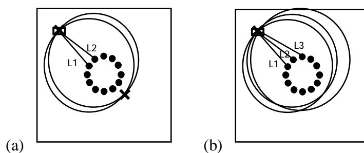
Rys.8. Lokalizacja uszkodzenia układem II czujników, (a) dwa przetworniki, (b) trzy przetworniki; □ – uszkodzenie zamodelowane, x – uszkodzenie zlokalizowane
