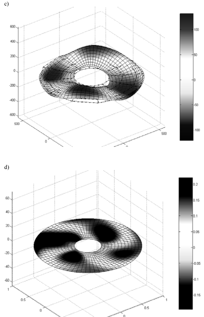
Rys. 8. Przykładowe wyniki analizy modalnej swobodnie zawieszonej tarczy silnika o mocy 2,2kW - forma odkształceń {a) i c)} i rozkład ciśnienia akustycznego w odległości 0,33m od powierzchni tarczy {b) i d)} dla częstotliwości: a) i b) 2700Hz, c) i d) 5400Hz.
