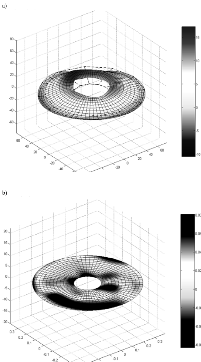
Rys. 8. Przykładowe wyniki analizy modalnej swobodnie zawieszonej tarczy silnika o mocy 2,2kW - forma odkształceń {a) i c)} i rozkład ciśnienia akustycznego w odległości 0,33m od powierzchni tarczy {b) i d)} dla częstotliwości: a) i b) 2700Hz, c) i d) 5400Hz.
