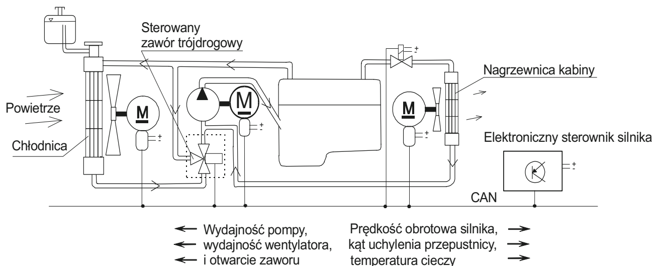
Rys. 8. Układ chłodzenia nowej generacji dla silnika samochodowego
