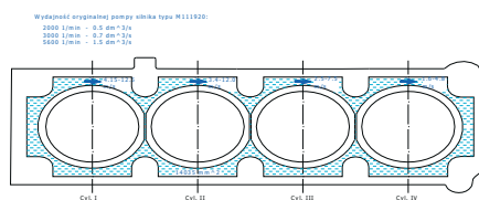
Rys. 4. Prędkości przepływu cieczy wokół tulei cylindrowych Fig. 4. Coolant velocities in engine block
