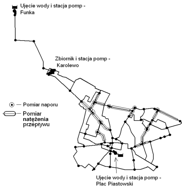
Rys. 2. Dopuszczalne miejsca alokacji urządzeń pomiarowych w sieci Chojnic Fig. 2. The allowable hydraulic sensor locations in Chojnice network
