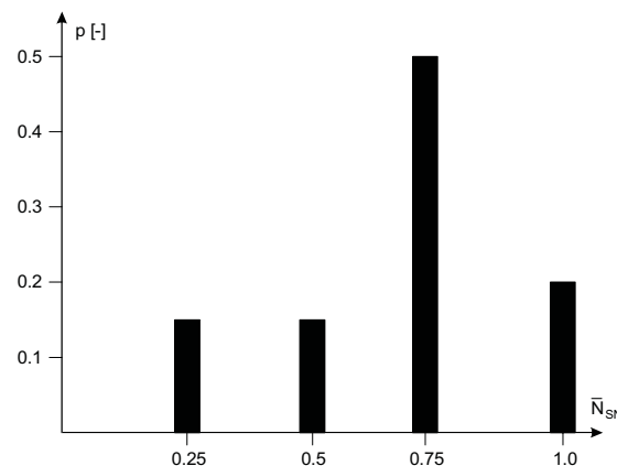
Rys. 3. Histogram rozkładów obciążeń silników głównych jednostek pływających pracujących w ciężkich warunkach E2 (przy \bar{n}_{SG} = idem ) i E3 (po krzywej śrubowej) [4-6]
