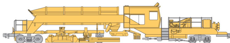
Rys. 15. Profilarka tłucznia [2]
